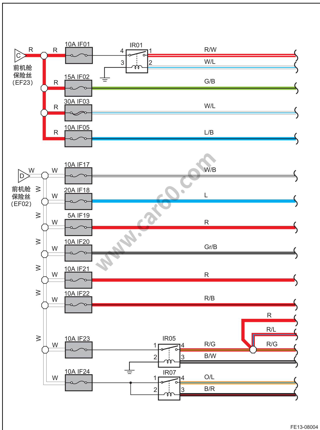
电源配电图 4
